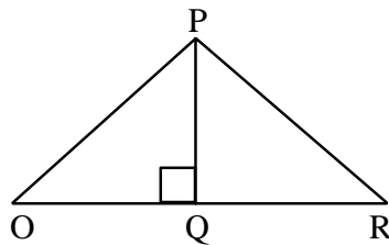
\Delta POR Gi \angle OPR = 90^\circ
