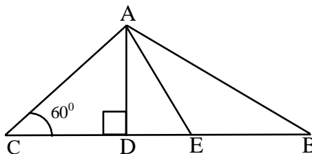
\Delta ABC Gi BC Gi gāv̄ēt̄ȳ E, AD = 4 t̄m.v̄g. Ges BC = 6 t̄m.v̄g.
